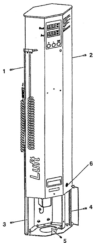
Slika 2: Shematski prikaz tlakomjera za gume tip AutoAir II s opisom pripreme za stavljanje uređaju u upotrebu
